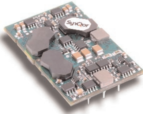
PQ60018QML15 Module
